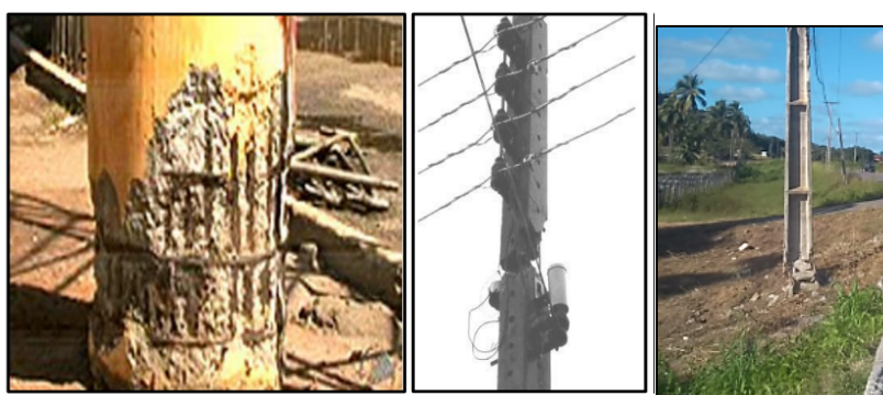
Foto 02 - Exemplo de base e topo de poste de concreto danificado.
